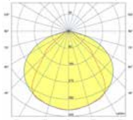
Systéo UNIT klar mit 90°-Optik
