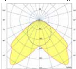
Systéo UNIT klar mit Batwing-Optik
